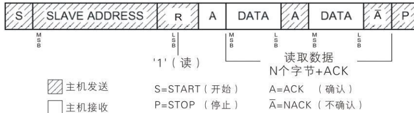
图 8: I2C 总线主机从从机接收数据的基本格式
